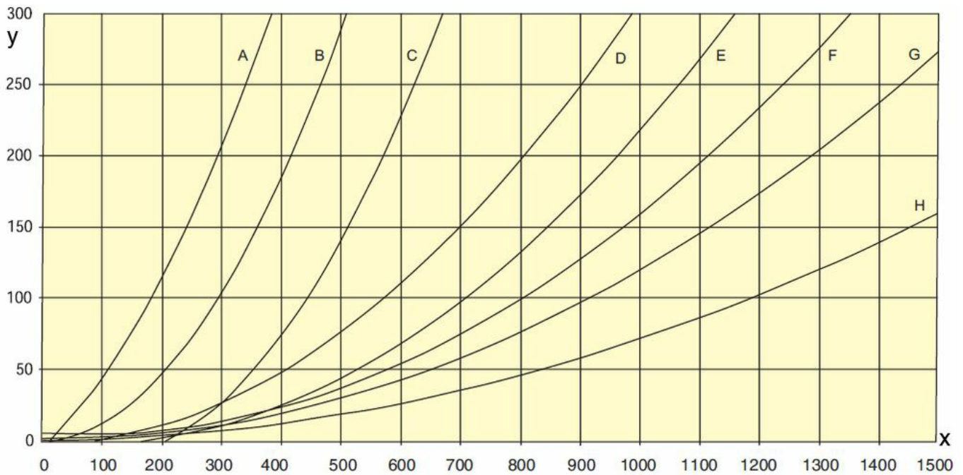
Y = Spadek ciśnienia Pa/m X = Wydajność m³/h A= Ø75 mm (3") na bębnie B= Ø75 mm (3") prosty C= Ø100 mm (4") na bębnie D=Ø125 mm (5") na bębnie E= Ø100 mm (4") prosty F= Ø150 mm (6") na bębnie G= Ø125 mm (5") prosty H= Ø150 mm (6") prosty
